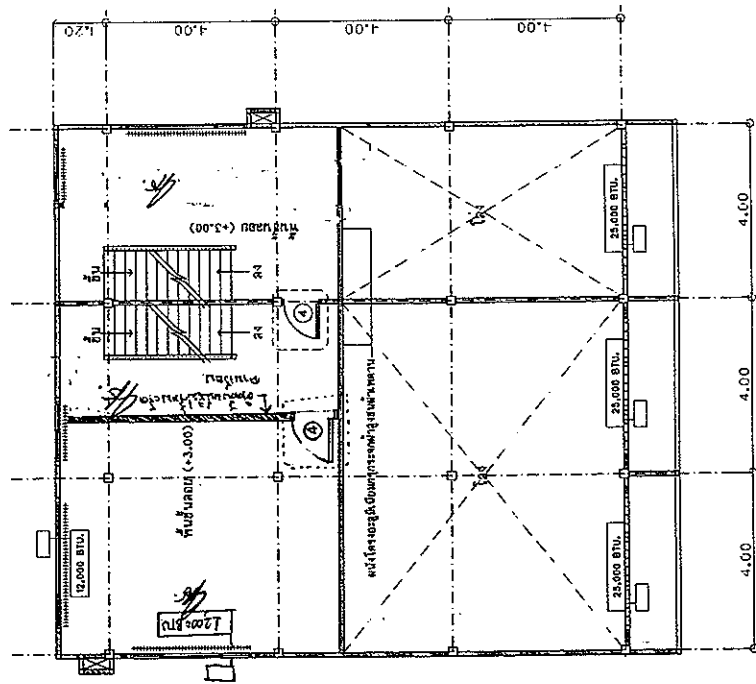
ผังชั้นลอย ขนาดรวม 1125
