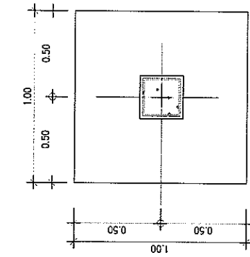
F1 PLAN SCALE 1:20
