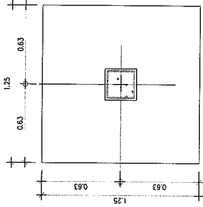
F2 PLAN SCALE 1:20
